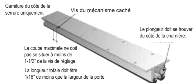
ILLUSTRATION 1 (Guide de coupe)
