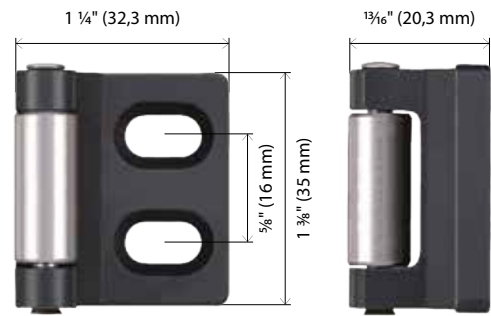
N° DXAS203 Gâche supérieure Pour DX2PV, DX2PW.
